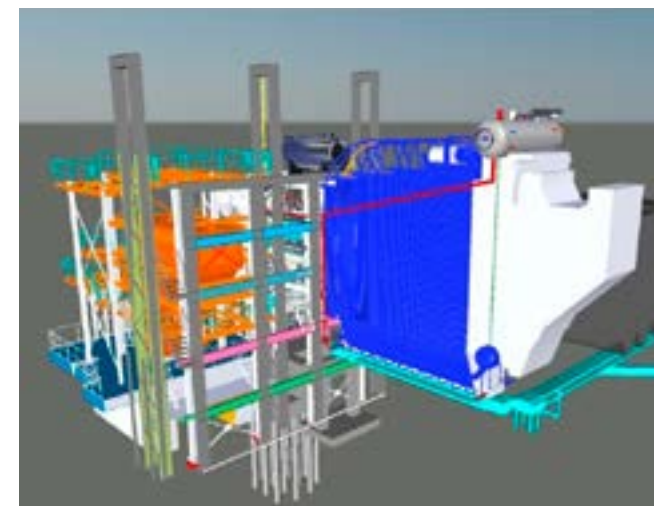
Maqueta Horno Volatilizador V
